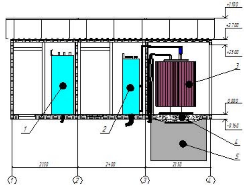
Разрез 1-1
